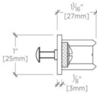
SIDE VIEW SCALE: 6"=1'-0"
