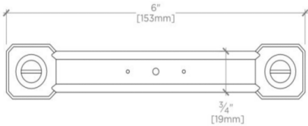
FRONT VIEW SCALE: 6"=1'-0"
