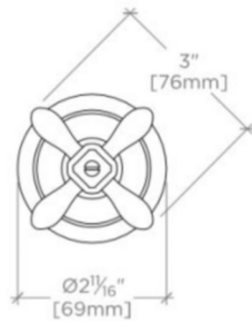
FRONT VIEW SCALE: 3"=1'-0"
