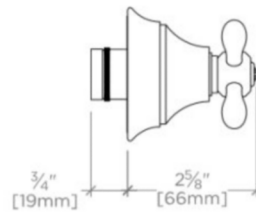
SIDE VIEW SCALE: 3"=1'-0"
