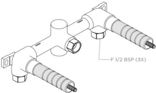
ISO VIEW SCALE: 3"=1'-0"
