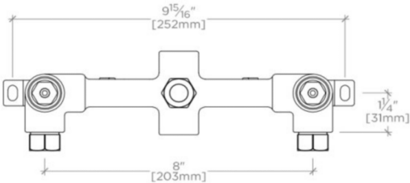
FRONT VIEW SCALE: 3"=1'-0"
