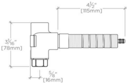
SIDE VIEW SCALE: 3"=1'-0"
