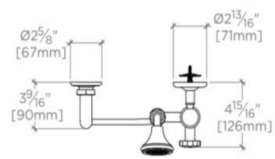
TOP VIEW SCALE: 1"=1'-0"
