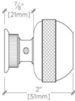
SIDE VIEW SCALE: 6"=1'-0"
