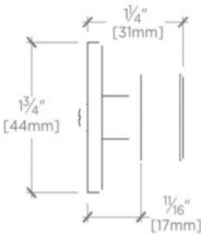
SIDE VIEW SCALE: 6"=1'-0"
