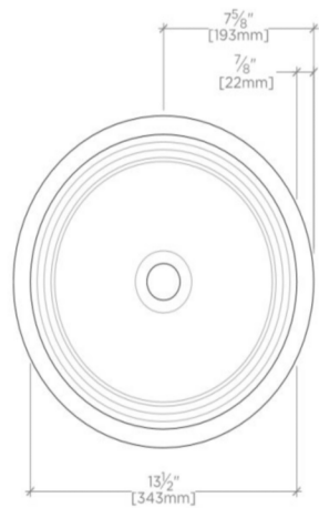
TOP VIEW SCALE: 1 1/2"=1'-0"
