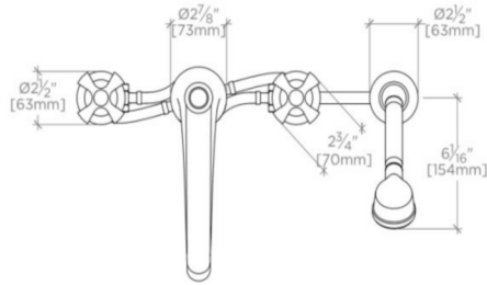
SCALE: 1/2"=1'-0"
