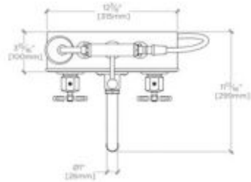
TOP VIEW SCALE: 5/16"=1'-0"
