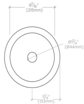
TOP VIEW SCALE: 1 1/2"=1'-0"
