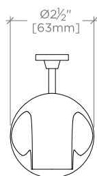
FRONT VIEW SCALE: 3"=1'-0"
