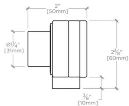
SIDE VIEW SCALE: 6"=1'-0"
