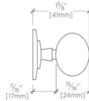
SIDE VIEW SCALE: 6"=1'-0"
