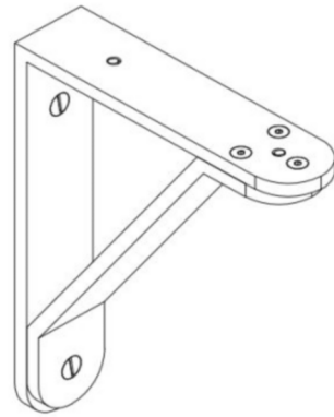
ISO VIEW SCALE: 3"=1'-0"
