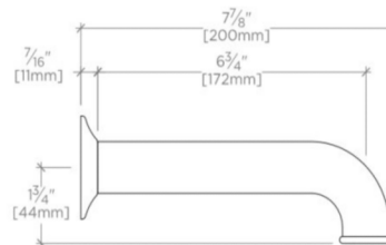
SIDE VIEW SCALE: 3"=1'-0"
