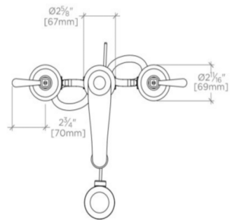
TOP VIEW SCALE: 1 1/2"=1'-0"
