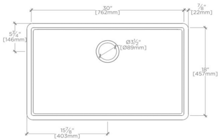
TOP VIEW SCALE: 1"=1'-0"
