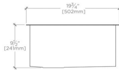
SIDE VIEW SCALE: 1"=1'-0"
