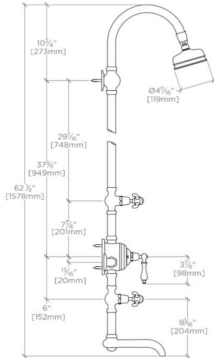
SIDE VIEW SCALE: 1"=1'-0"
