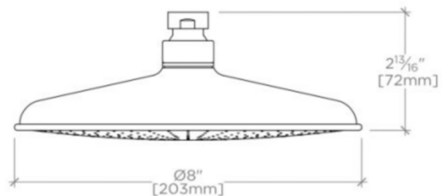
SIDE VIEW SCALE: 3"=1'-0"
