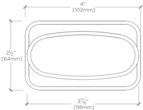
FRONT VIEW SCALE: 6"=1'-0"
