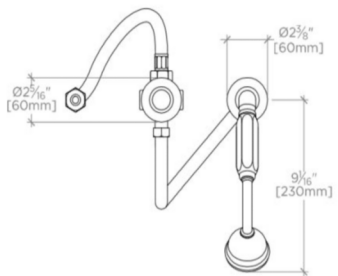
TOP VIEW SCALE: 1 1/2"=1'-0"
