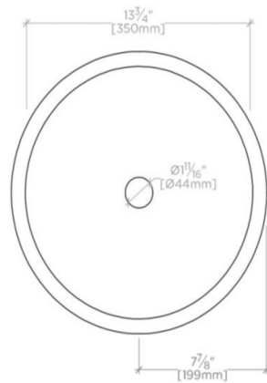
TOP VIEW SCALE: 1/2"=1'-0"
