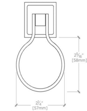
FRONT VIEW SCALE: 6"=1'-0"
