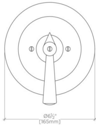
FRONT VIEW SCALE: 3"=1'-0"
