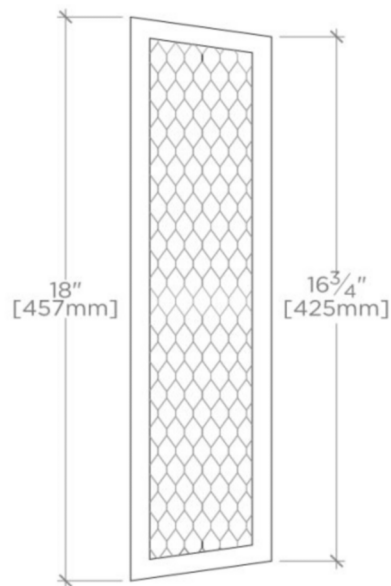
SIDE VIEW SCALE: 2"=1'-0"
