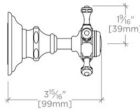
SIDE VIEW SCALE: 3"=1'-0"
