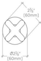
FRONT VIEW SCALE: 3"=1'-0"
