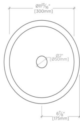
TOP VIEW SCALE: 1 1/2"=1'-0"
