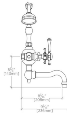
SIDE VIEW SCALE: 1½"=1'-0"
