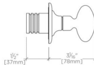
SIDE VIEW SCALE: 3"=1'-0"
