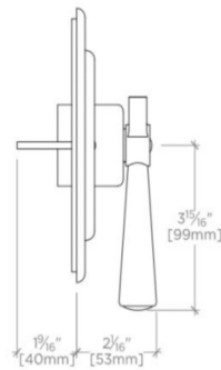
SIDE VIEW SCALE: 3"=1'-0"
