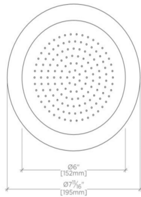
CEILING VIEW SCALE: 3"=1'-0"
