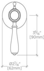
FRONT VIEW SCALE: 3"=1'-0"
