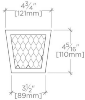
TOP VIEW SCALE: 2"=1'-0"
