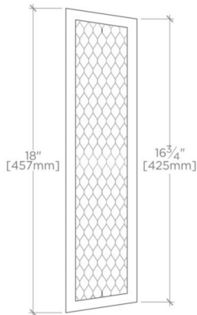
SIDE VIEW SCALE: 2"=1'-0"
