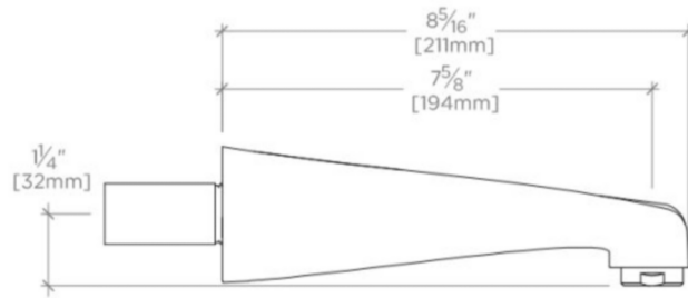
SIDE VIEW SCALE: 3"=1'-0"
