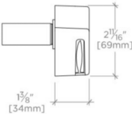
SIDE VIEW SCALE: 3"=1'-0"
